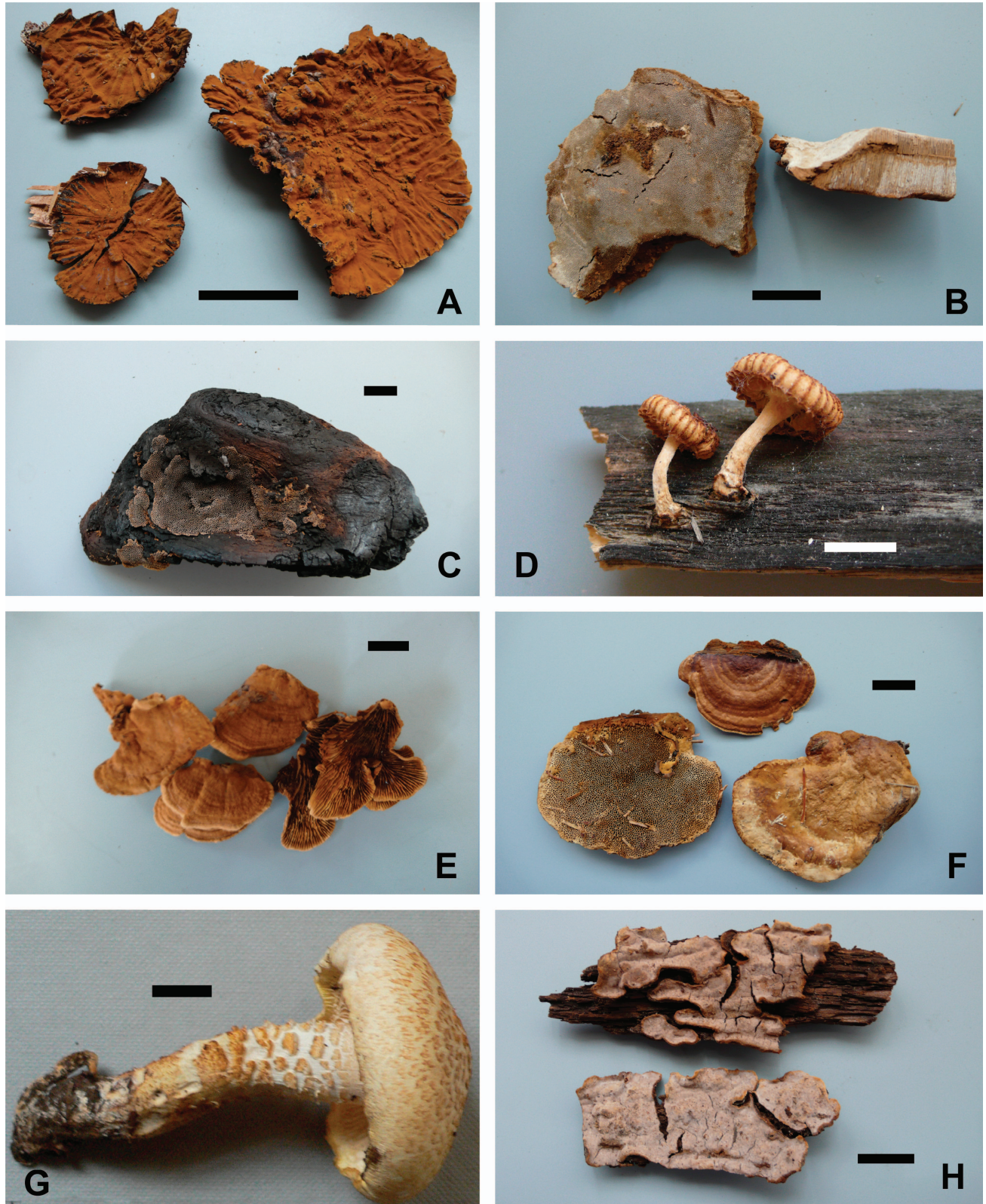
FIG. 1. Fruiting body diversity in Gloeophyllales and Donkioporia expansa (Polyporales). A. Boreostereum radiatum (Peck) Parmasto DAOM 160898. B. Donkioporia expansa (Desm.) Kotl. & Pouzar AN028794. C. Gloeophyllum carbonarium (Berk. & M.A. Curtis) Ryvarden AN010068. D. Heliocybe sulcata (Berk.) Redhead & Ginns IBUG 9930. E. Gloeophyllum sepiarium (Wulfen) P. Karst. AN028562. F. Gloeophyllum protractum (Fr.) Imazeki AN032340. G. Neolentinus lepideus (Fr.) Redhead & Ginns RGS-DSH s.n. H. Veluticeps berkeleyi Cooke SD62-6-4. Bars = 1 cm.
